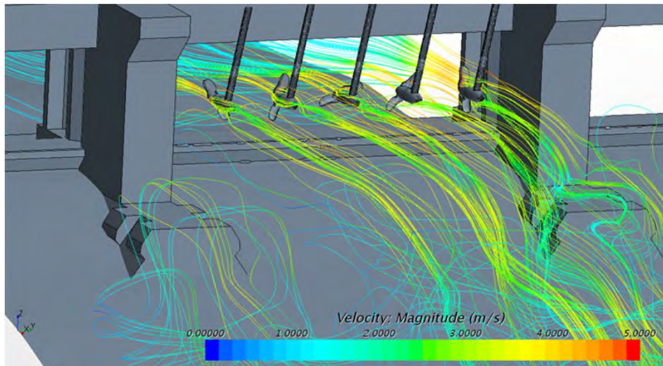
CFD model Roompot 08 met 5 turbines T200
