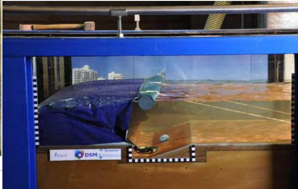
DYNEEMA tsunami barrier
